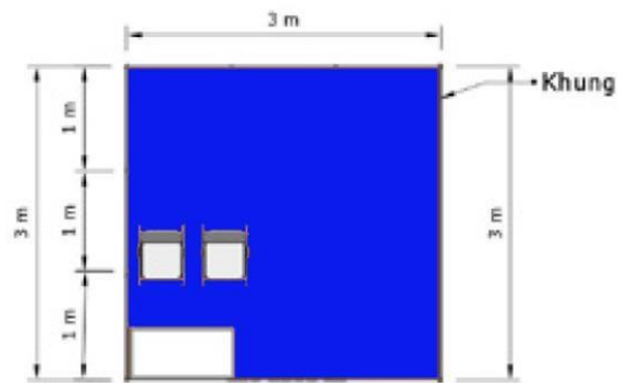
MẶT BẰNG
