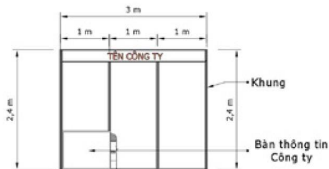
MẶT ĐỨNG
